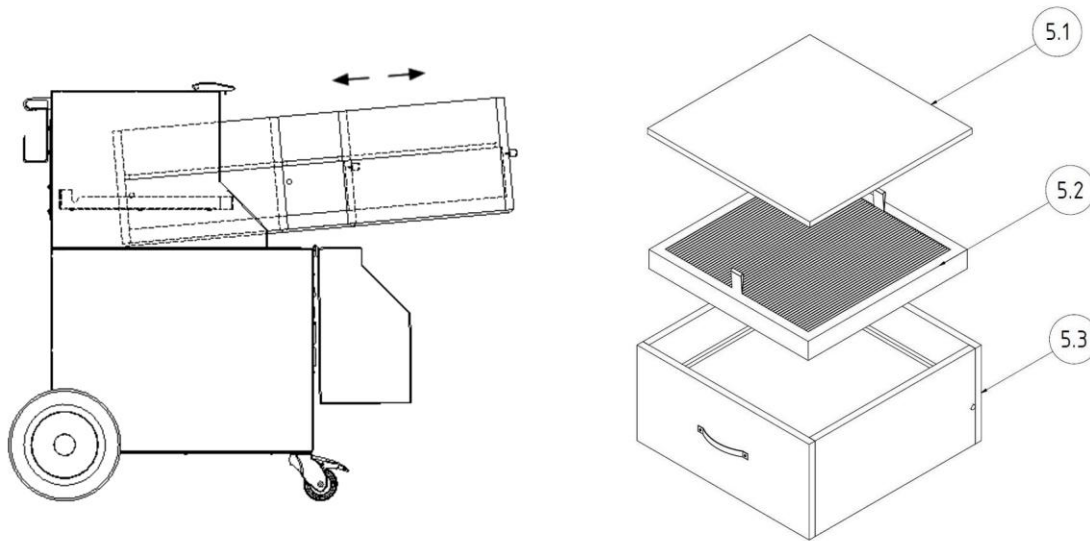
Abb. 4: Filterwechsel
